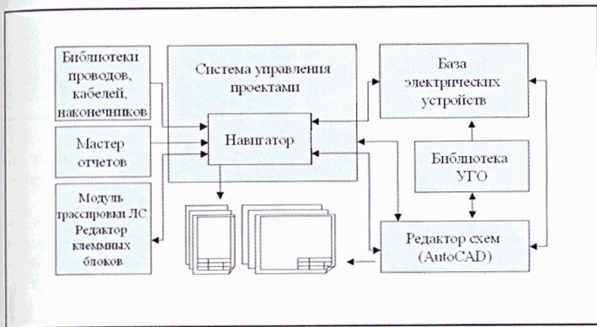
↑ Структурная схема ElectricCS 5.0
