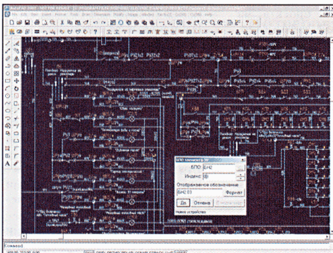
↑ Редактор схем
